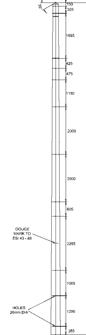
14 METRE POLE FABRICATION
